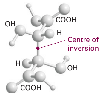
3 Meso-tartaric acid, \text{HOOCCH(OH)CH(OH)COOH}
